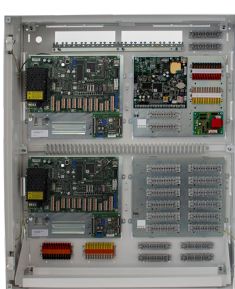
Gehäusetyp S110
